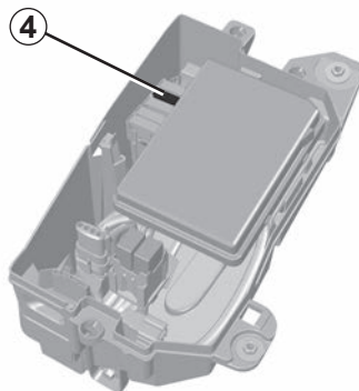
Fusible 4 : coupure circuit GPL.
